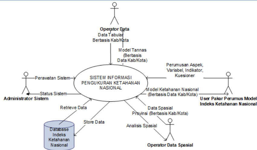
Gbr 4. Context Diagram Aplikasi Pengukuran Indeks Ketahanan Nasional
